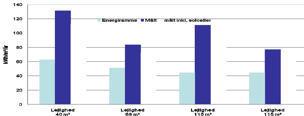
Figur 73, Peter Weitzmann, COWI søjlediagram visende beregnet og målt energiforbrug i kWh pr.m 2 pr. år
