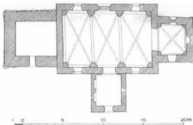
Fig. 2. Haldagerlille. Plan. 1:300. Maalt af Aage Rousell 1931.
