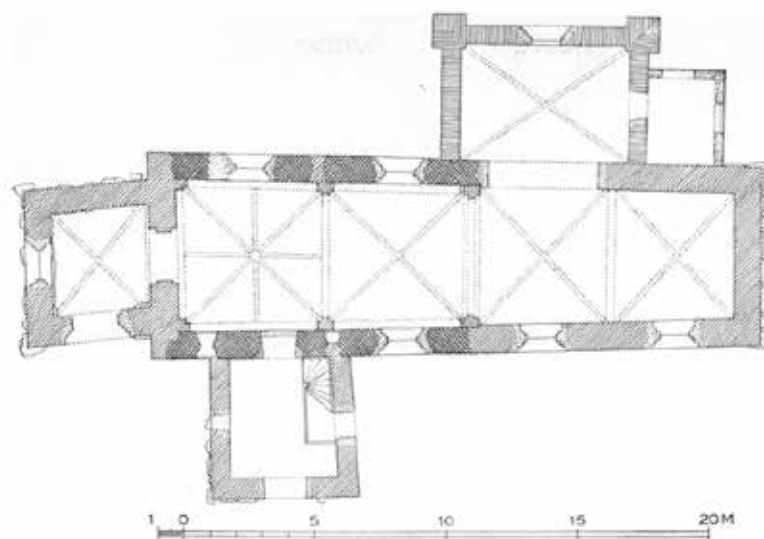
Fig. 2. Venslev. Plan. 1:300. Maalt af Arne Nystrom 1928.
