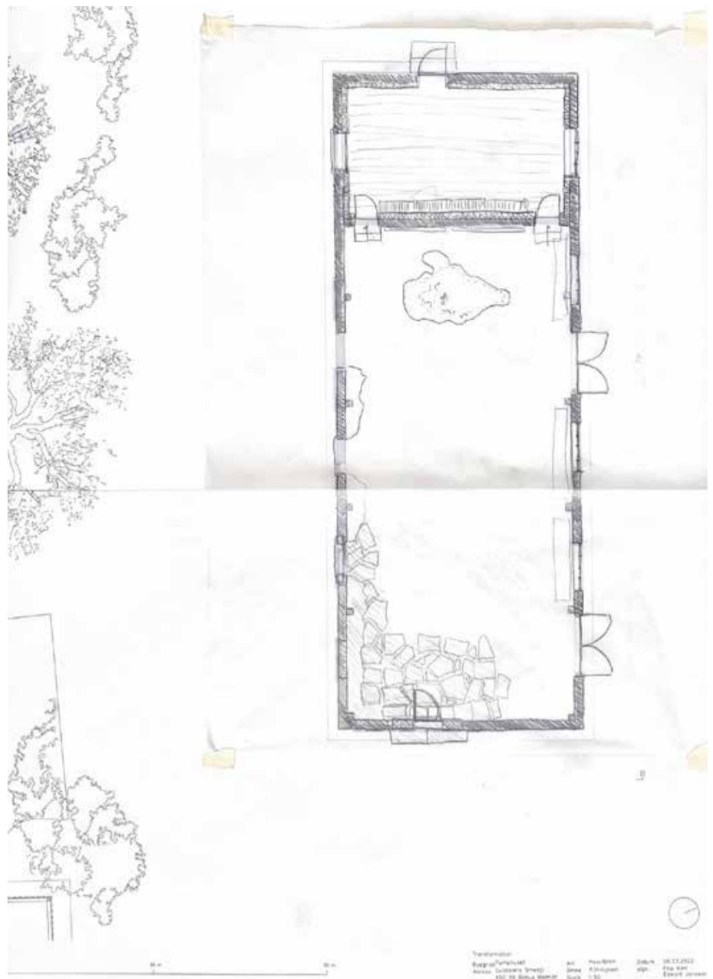
Pumphuset Planskiss
