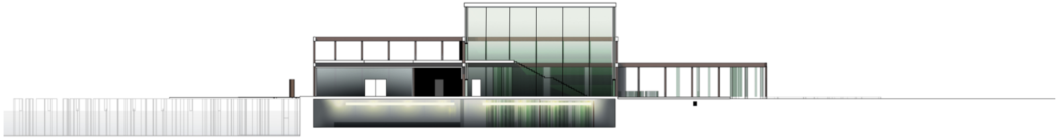
Snitt i Semiboks - S 1:200
