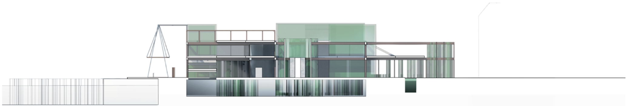
Snitt i offentlig sfære - S 1:200
