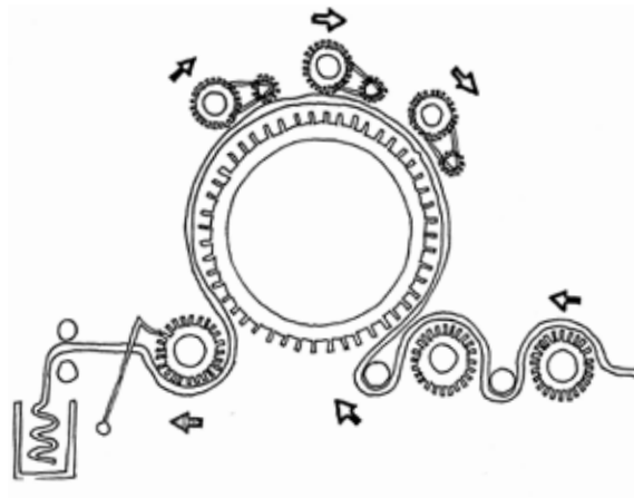
Meknisert kardemaskin
