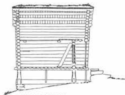
LANGSNITT MOT VEST
