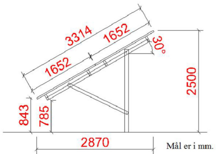
Figur 2.2.1 Tegning af anlægget
